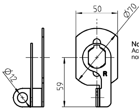
Accessori per lucchetto in acciaio polverizzato nero
