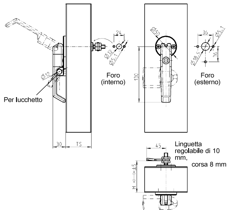
Fissaggio con rivetti
