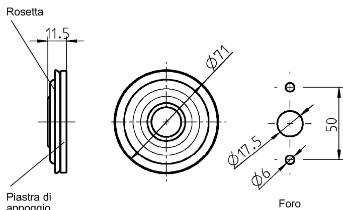
Rosetta in acciaio zincato
