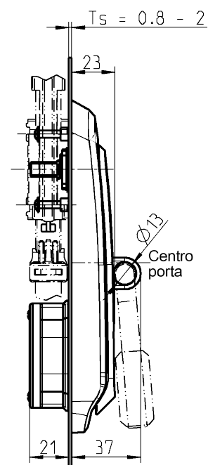
Maniglia girevole lucchettabile con coperchio e per serratura per aste
