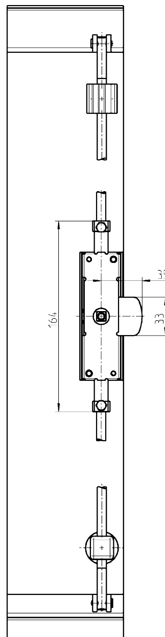
Disegno della versione destra
