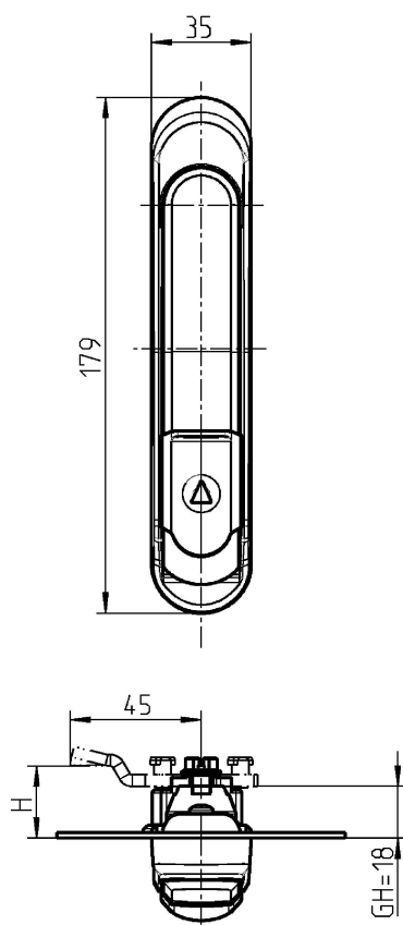
Maniglia girevole con coperchio e adattatore per linguetta
