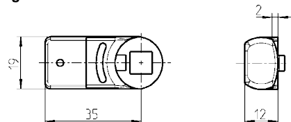
*Versione 3 Linguetta per aste per 3 punti di chiusura
