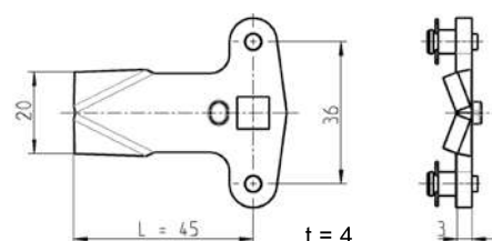
*Versione 3 Linguetta per aste per 3 punti di chiusura
